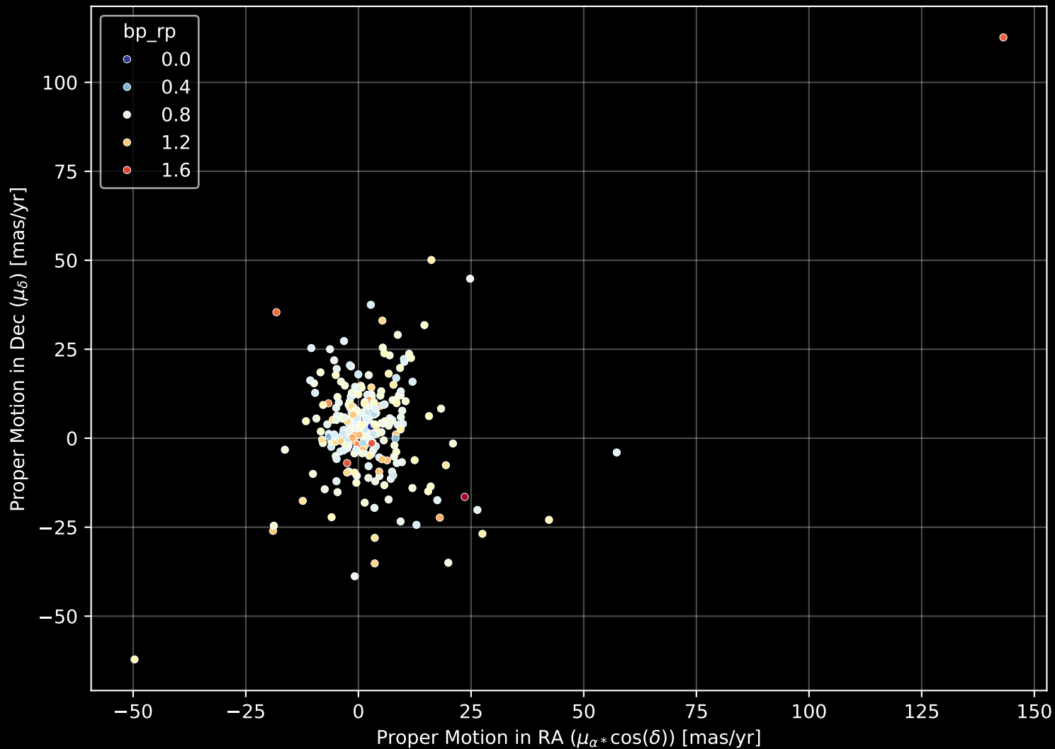
GALAH DR4 Field: [1474] Proper Motion Diagram (n= 284)
