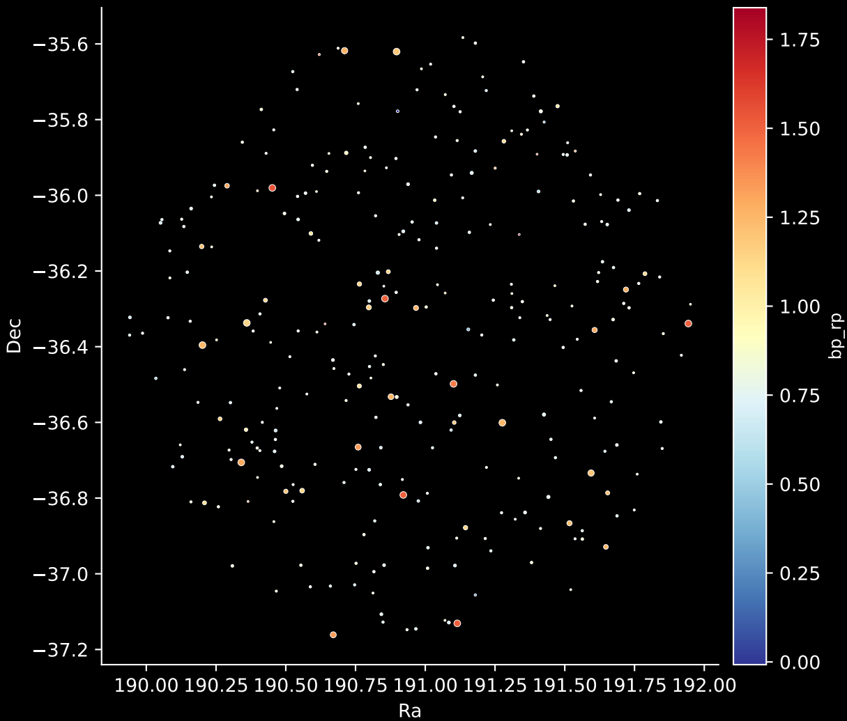
GALAH DR4 Field: [1474] Stars: 284
