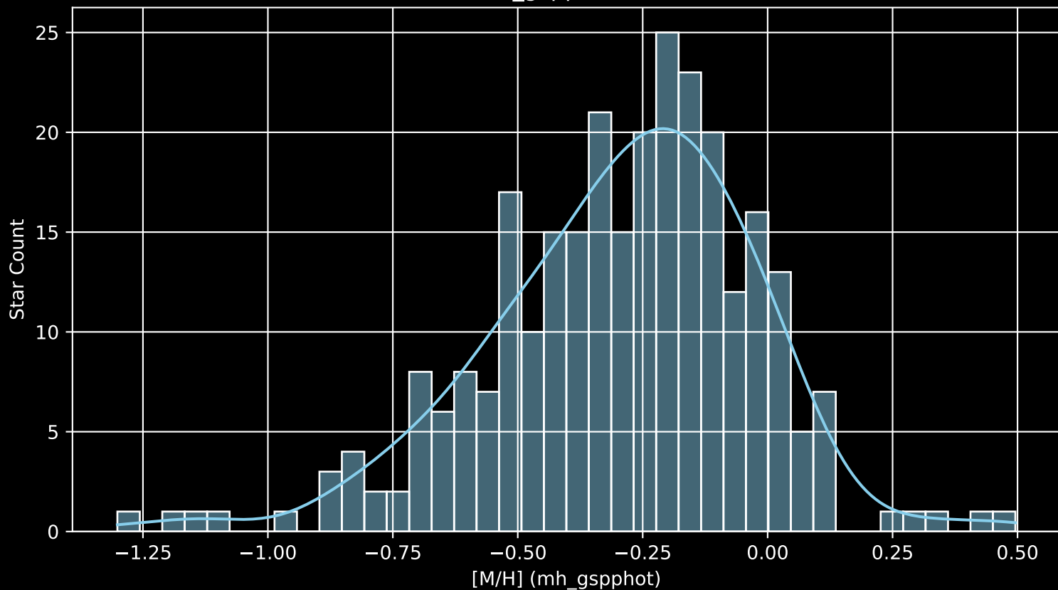
GALAH DR4 Field: [1474] [M/H] (mh_gspphot) (n= 284)
