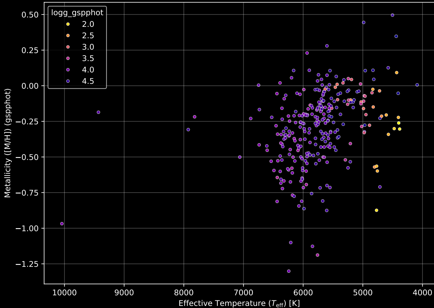
GALAH DR4 Field: [1474] Stellar Population Parameters (n= 284)
