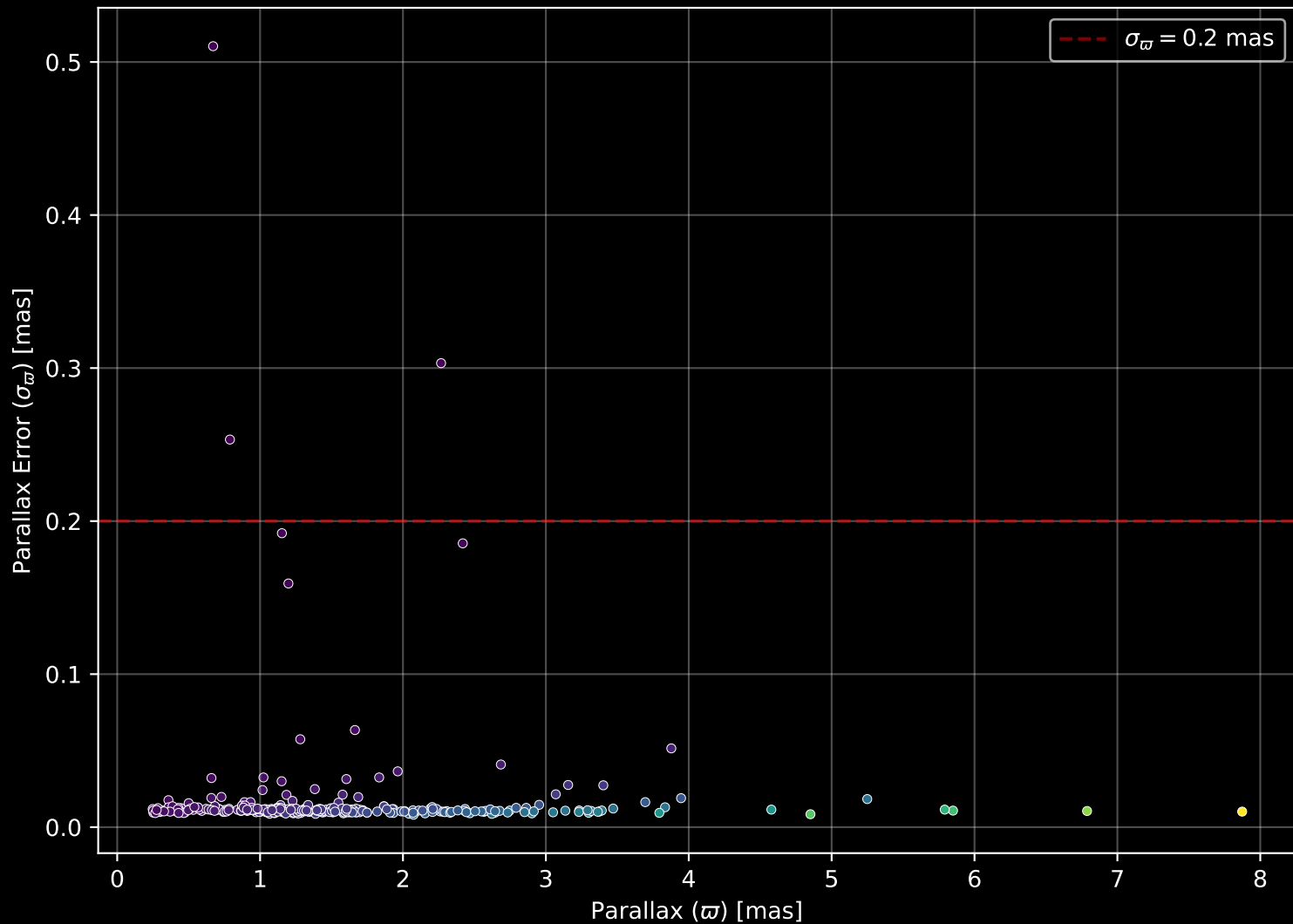
GALAH DR4 Field: [1474] Parallax Quality (n= 284)
